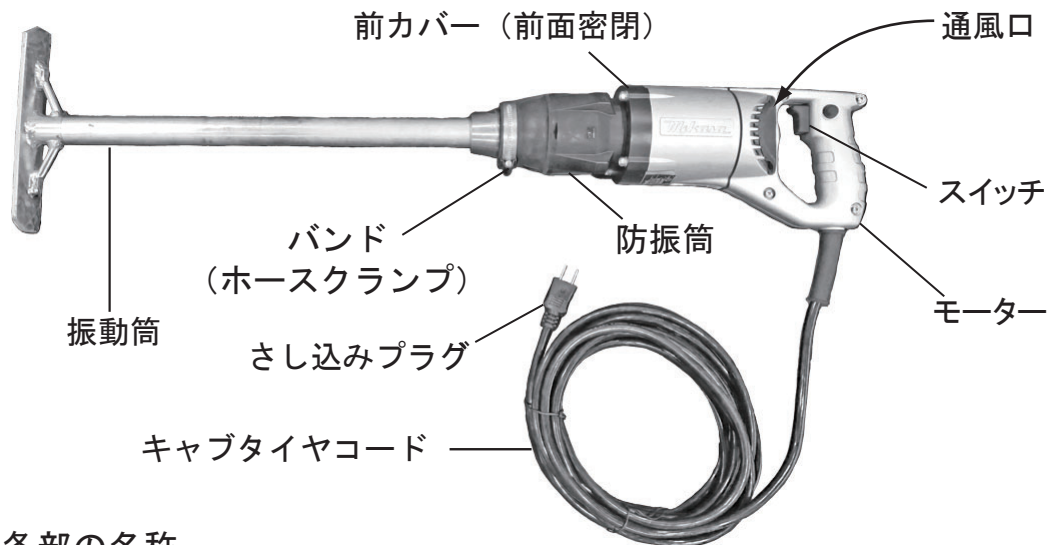
図 1 : 各部の名称
